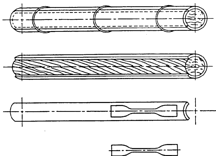
Figure B.2 – Préparation des éprouvettes en forme d'haltère après vieillissement
